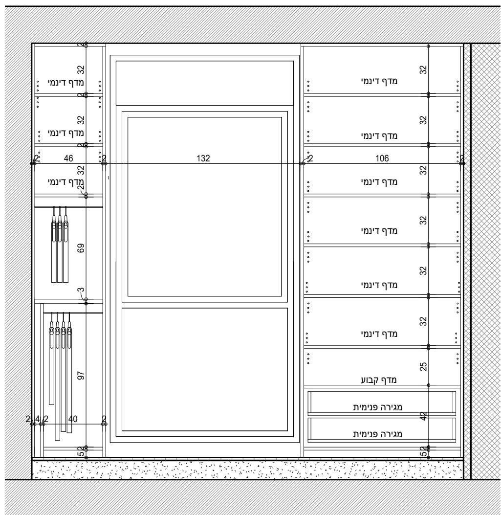
נ-4: חזית פתוחה ק.ג.מ: 1:25
