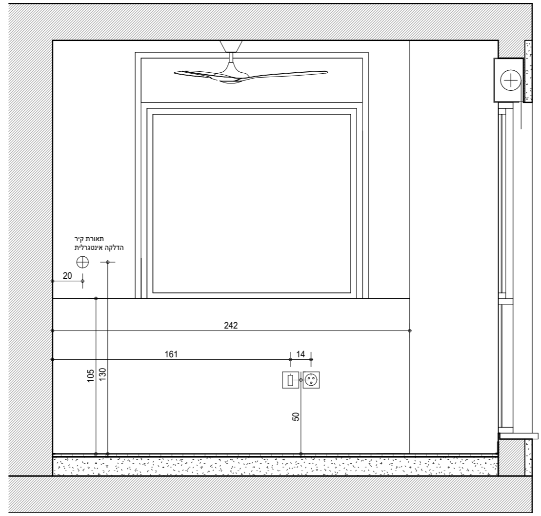
נ-3 : חזית 1 ק.ג. מ: 1:25
