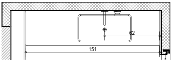
נ-12: תכנית ק.ג.מ: 1:25
