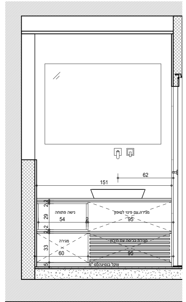
נ-12: חזית ק.ג.מ: 1:25
