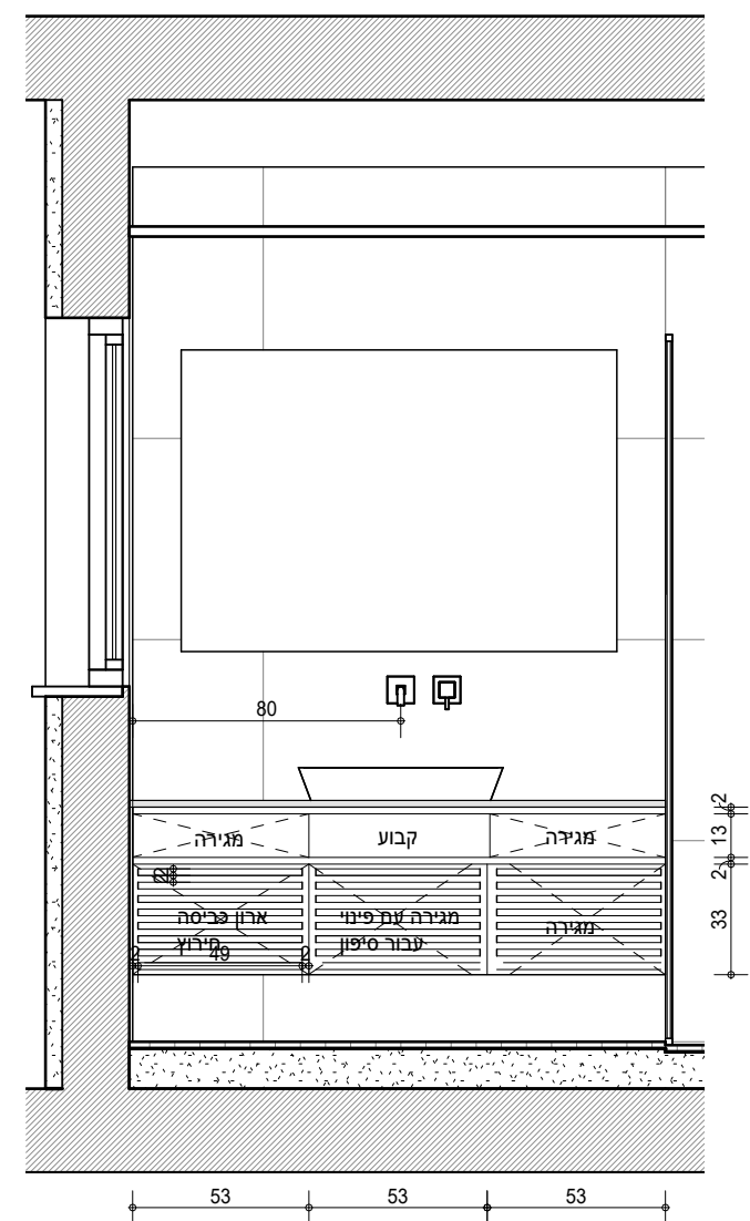
נ-7: חזית ק.ג.מ: 1:25
