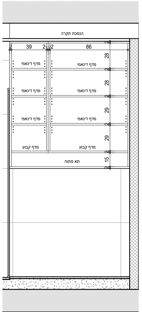
כ-11: חזית פתוחה ק.ג.מ: 1:25
