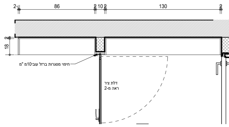
נ-13 תכנית ק.נ.מ. 1:25
