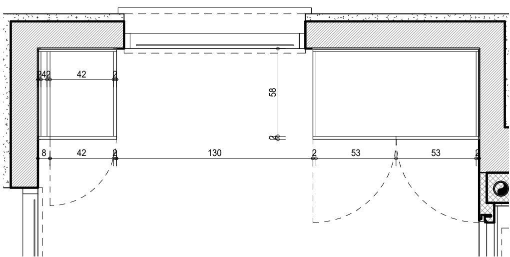
נ-4: תכנית ק.ג.מ: 1:25
