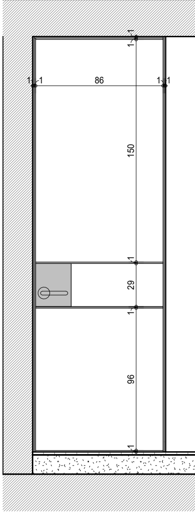
נ-6: חזית ק.ג.מ: 1:25
