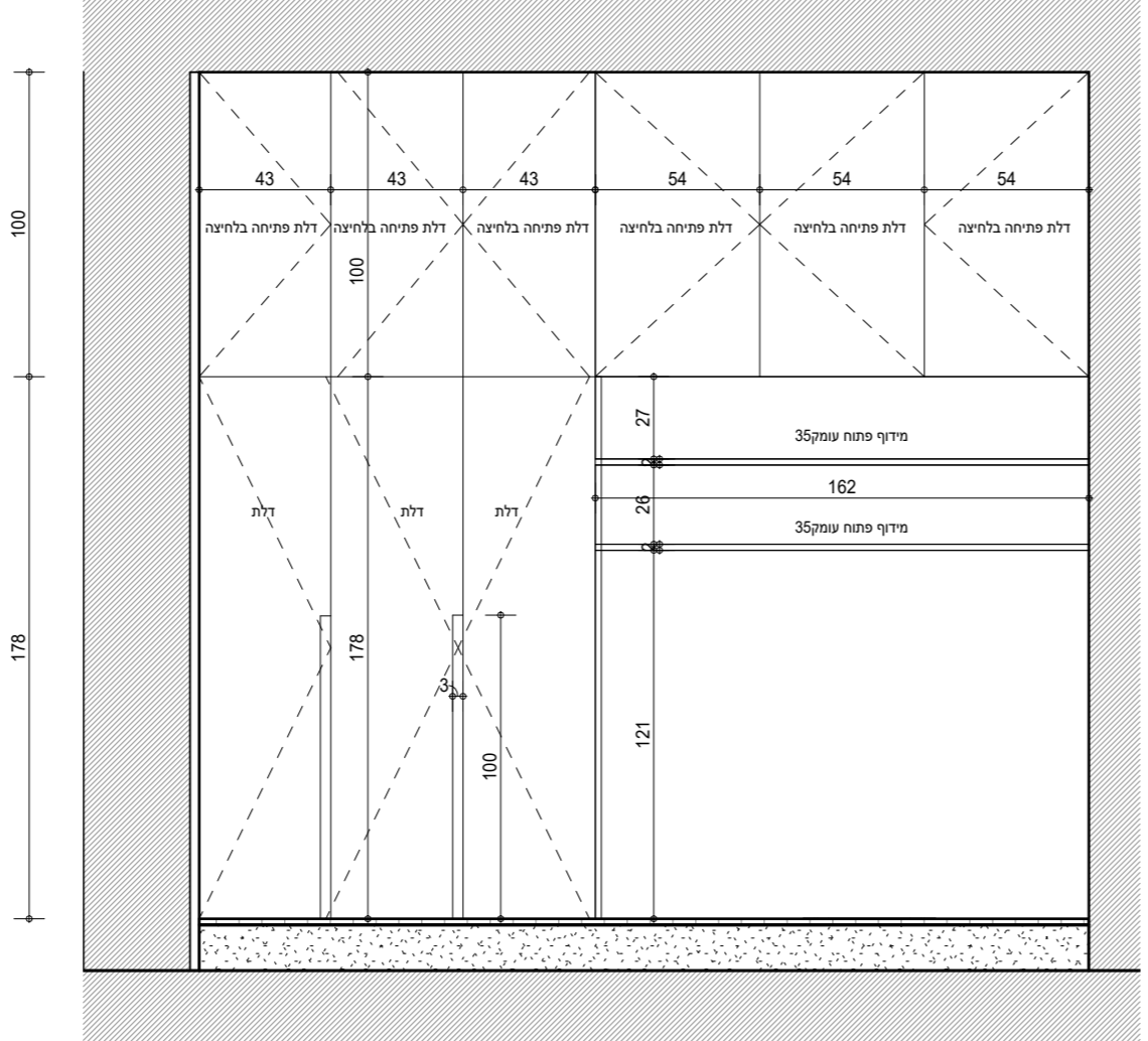
8-נ חזית 1:25, ק.נ.מ.
