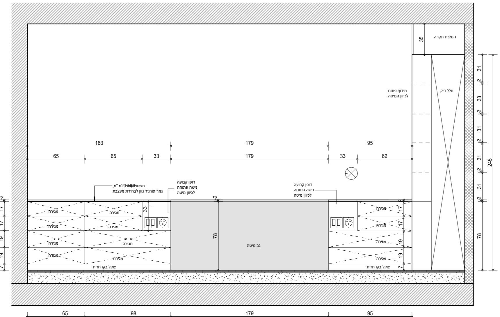
נ-9 חזית ק.ג.מ. 1:25
