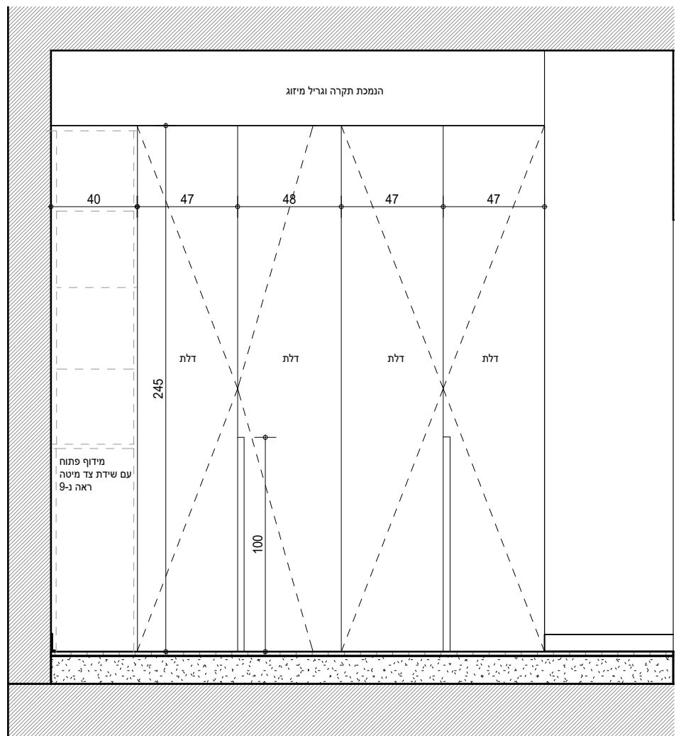
10-נ חזית ק.ג.מ. 1:25
