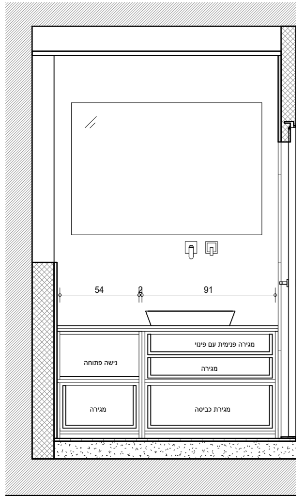
נ-12: חזית פתוחה ק.ג.מ: 1:25
