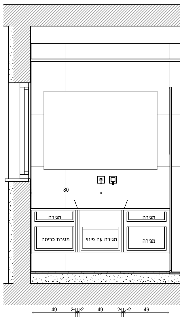
נ-7: חזית פתוחה ק.ג.מ: 1:25
