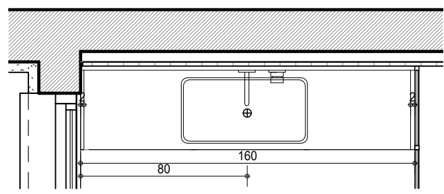
נ-7: תכנית ק.ג.מ: 1:25
