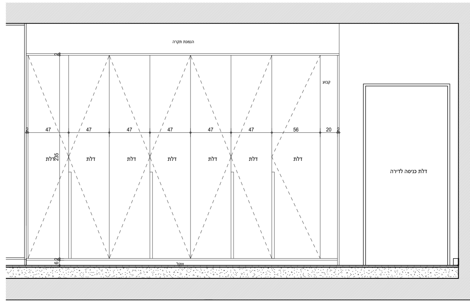
נ-1: חזית ק.ג.מ. 1:25
