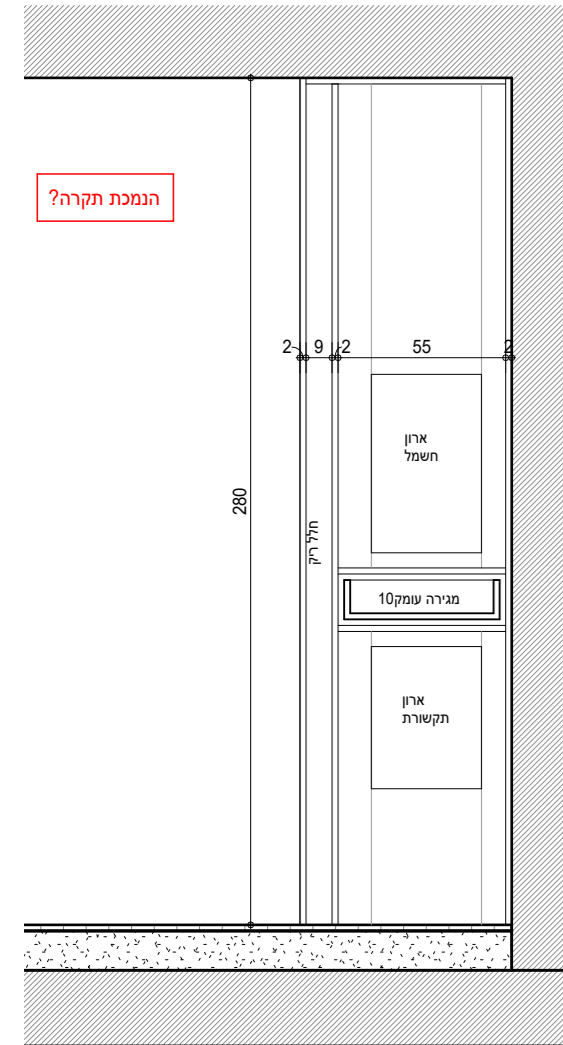
נ-6: חזית פתוחה ק.ג.מ. 1:25
