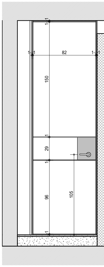
מ-2: חזית ק.ג.מ: 1:25
