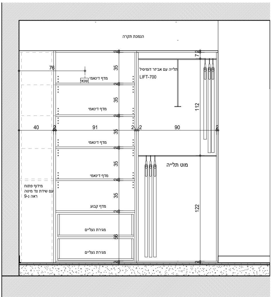
10-נ חזית פתוחה ק.ג.מ. 1:25
