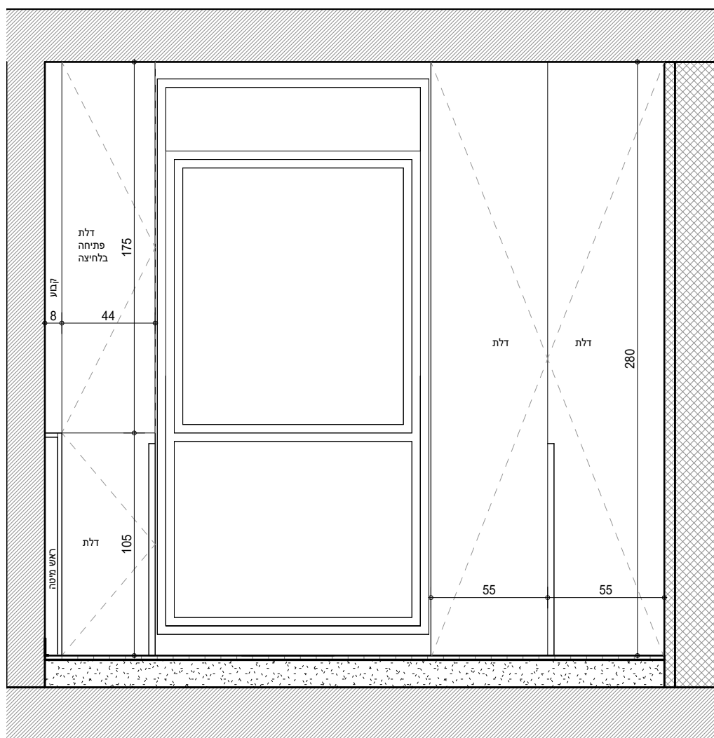
נ-4: חזית ק.ג.מ: 1:25
