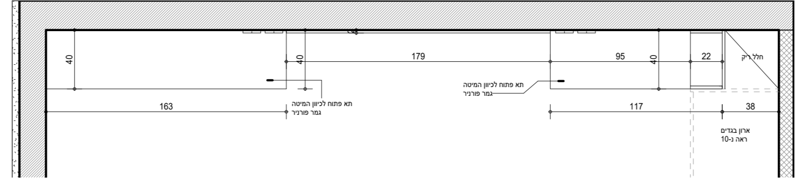
נ-2 תכנית ק.ג.מ. 1:25
