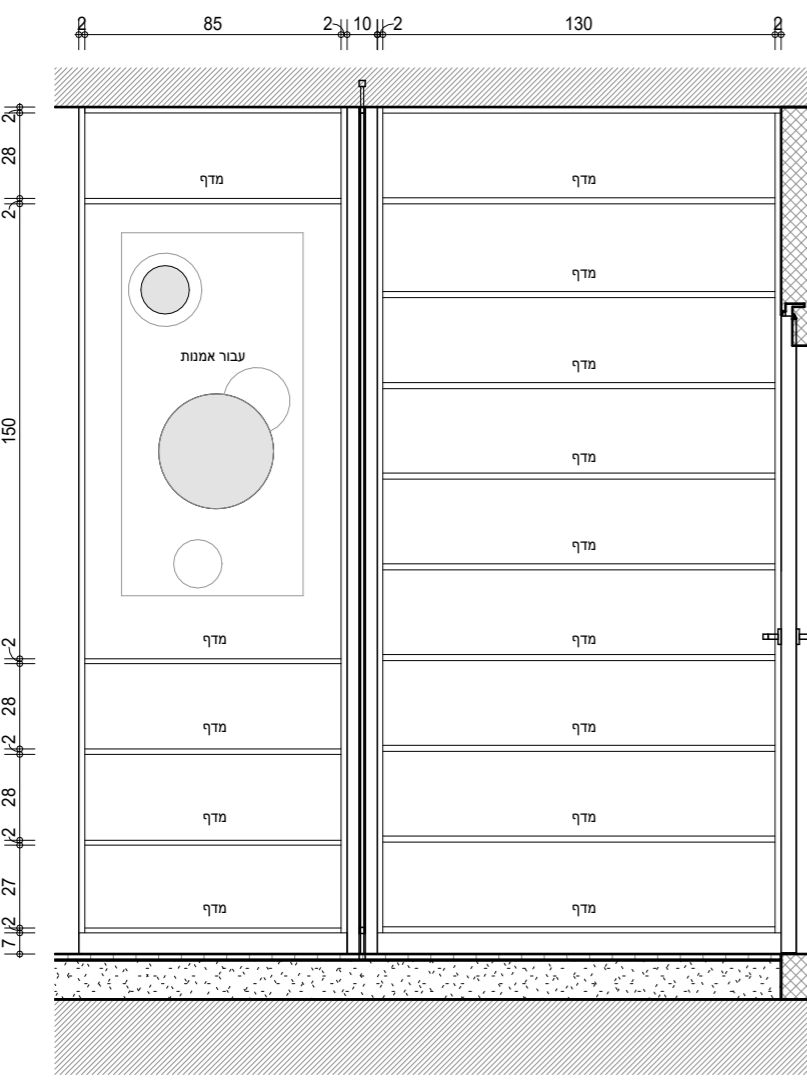
נ-13 חזית ק.נ.מ. 1:25
