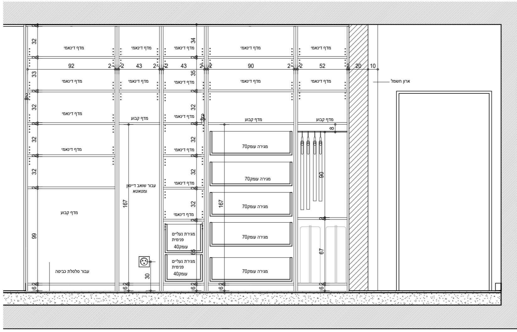
נ-1: חזית פתוחה ק.ג.מ. 1:25
