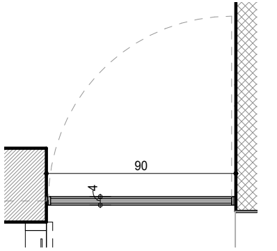
מ-3: תכנית ק.ג.מ: 1:25
