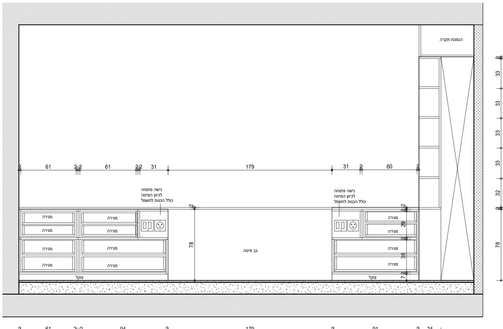
נ-2 חזית פתוחה ק.ג.מ. 1:25
