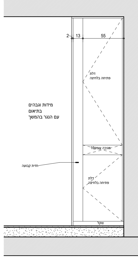
נ-1: חזית ק.ג.מ. 1:25
