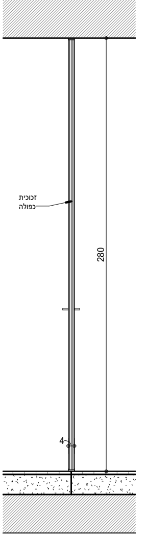
נ-6: חזית פתוחה ק.ג.מ: 1:25
